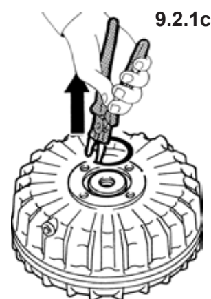
GIUNTI GRANDEZZA 75/85
