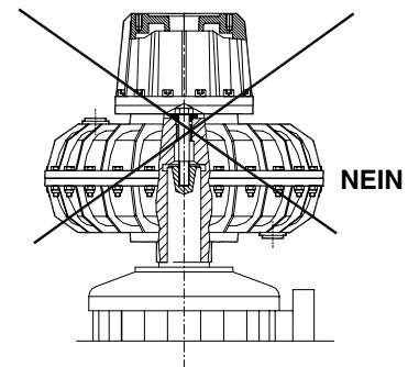
VERTIKALE WELLE MIT OBEN LIEGENDER VERZÖGERUNGSKAMMER
