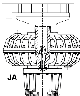
VERTIKALE WELLE MIT UNTEN LIEGENDER VERZÖGERUNGSKAMMER
